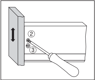
上下調整 ±2mm
