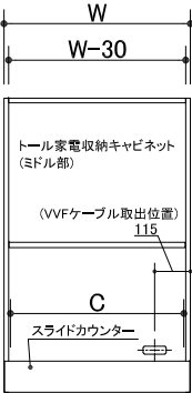
トール家電収納キャビネット(ミドル部)
